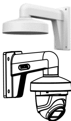
DS-1272ZJ-110-TRS Mocowanie ścienne
