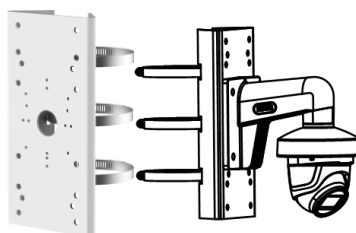
DS-1275ZJ-SUS Mocowanie słupowe
